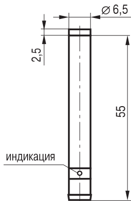
Габаритный чертёж
